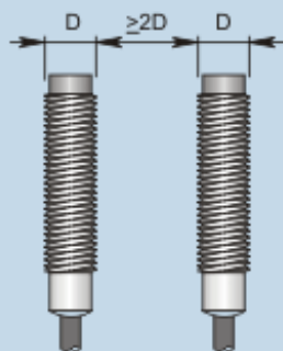
Montaggio affiancato
